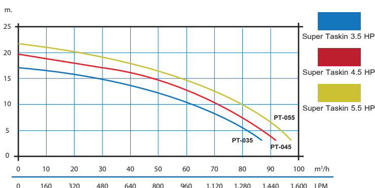
กราฟแสดงประสิทธิภาพอัตราการไหล
